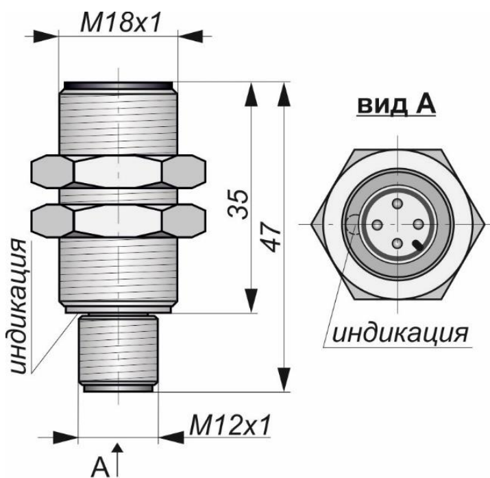
Габаритный чертеж
